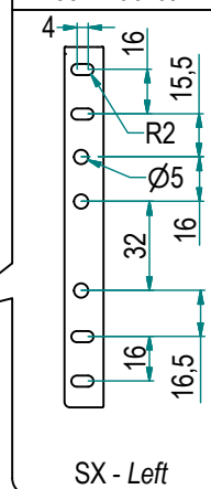
Squadretto Anta Door Bracket
